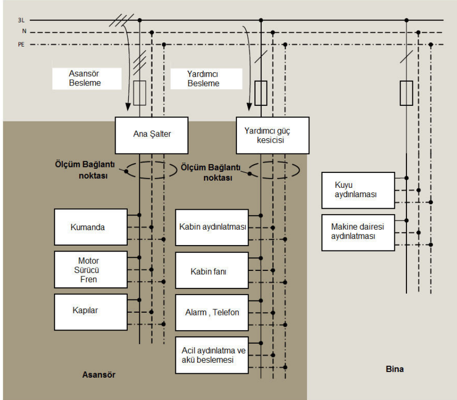
Şekil-1 Ölçüm bağlantı noktaları
