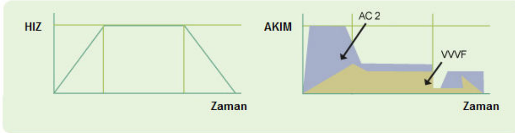
Şekil-7 AC-2 AC-VVVF seyahat akım grafiği
